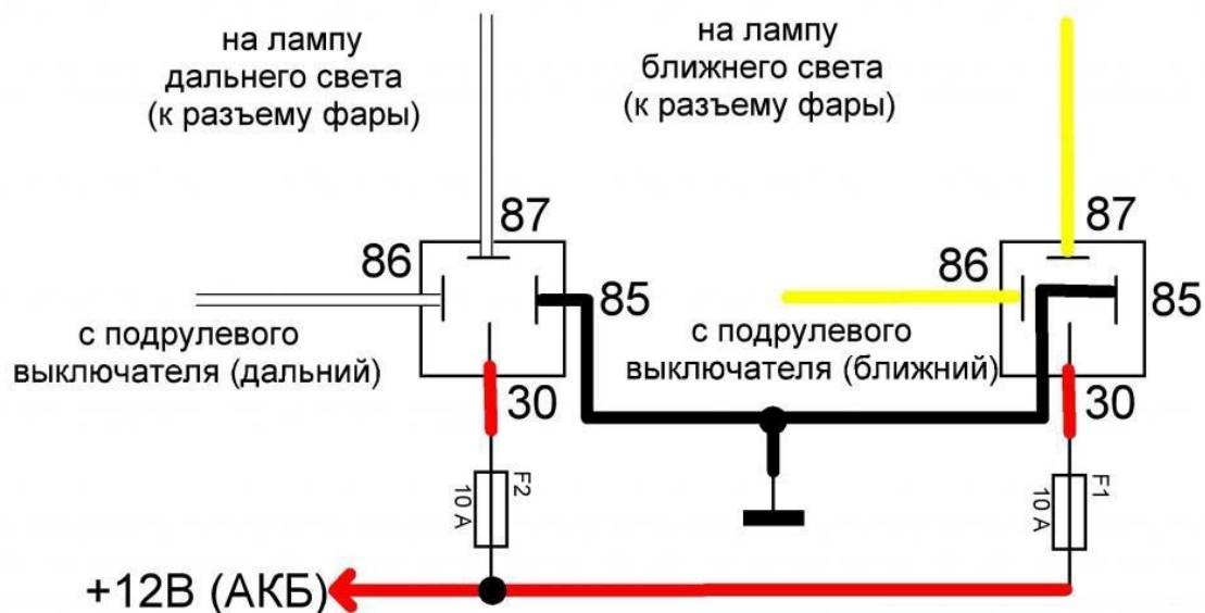
Рисунок 1. Схема подключения фар головного света.
